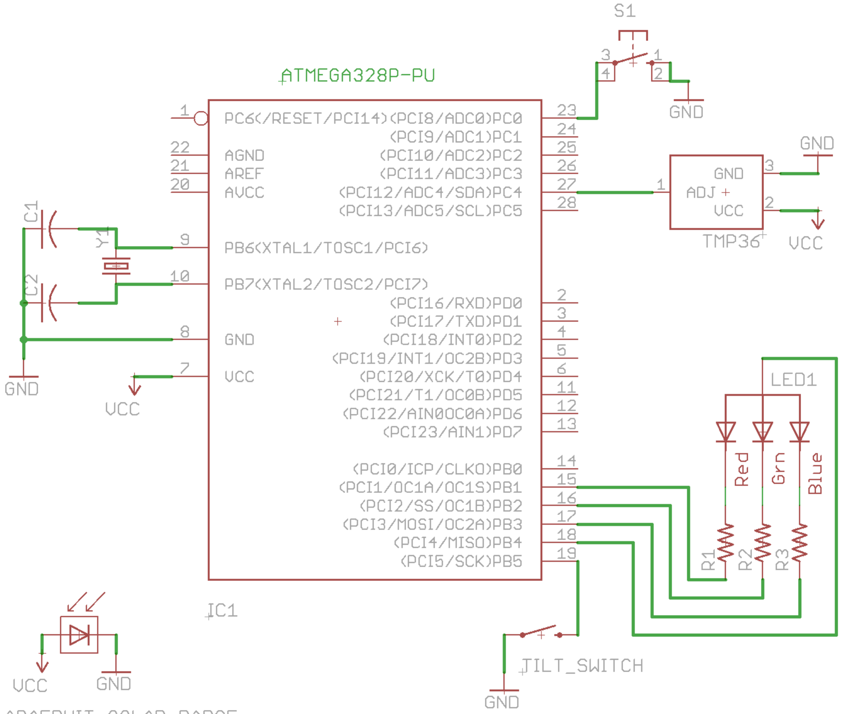
ADAFRUIT_SOLAR_BADGE
